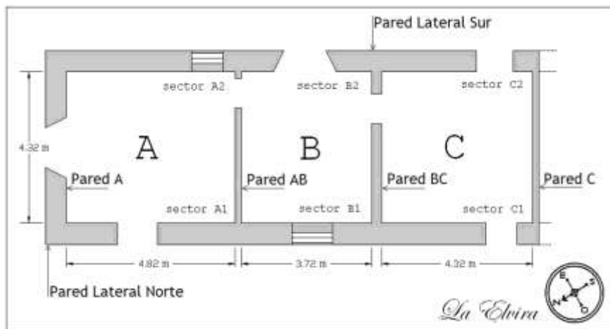
Figura 3. Croquis de la vivienda que incluye la denominación de los sectores tal como se utilizó durante el trabajo de campo.
